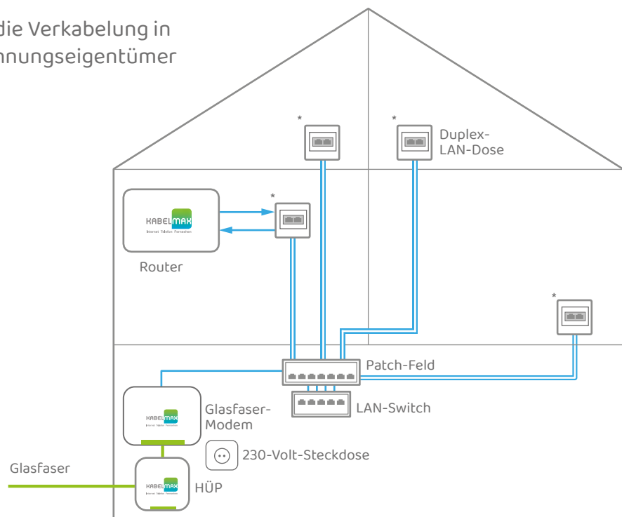
HÜP und Glasfaser-Dose sind im Einfamilienhaus (EFH) eine Komponente.
